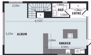
STUEPLAN
